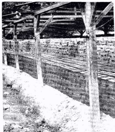
7) 壓實後的磚塊，置於四面通風的棚下風乾。
