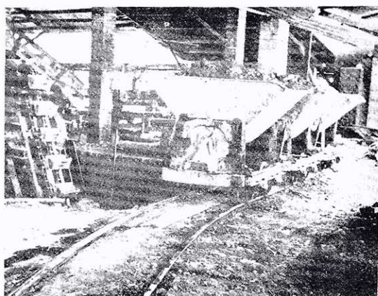
2) 由山上採來的紅泥，由運輸帶運到練泥機，練成泥膠。
