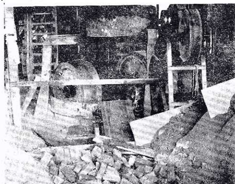
3) 磨泥機把紅泥、沙礫及碎磚磨成粉末，以便滲水拌合，成為泥漿。
