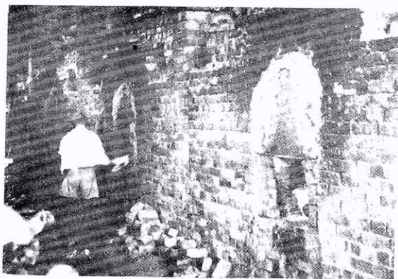
9) 窖口用泥密封，裡面火勢正烈，外頭熱氣迫人。
